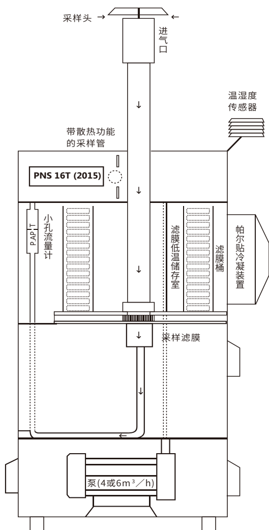
产品结构图
