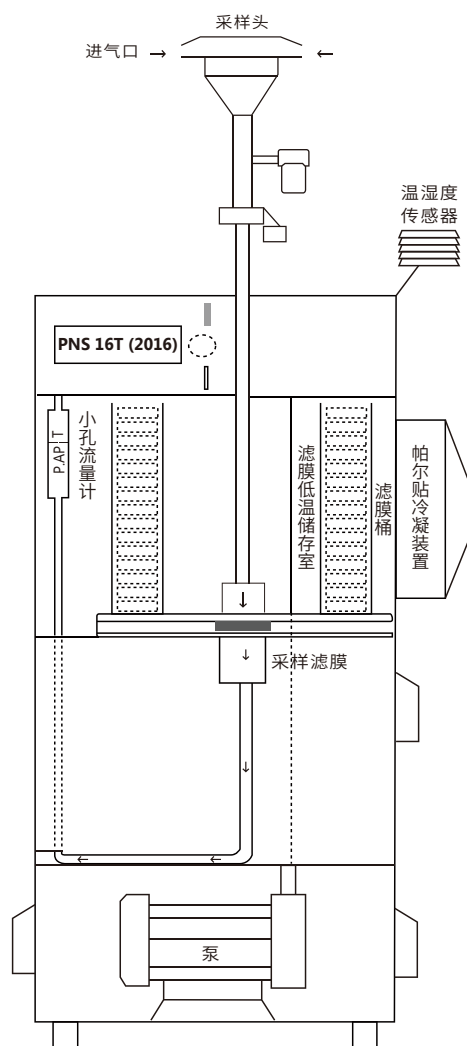
产品结构图
